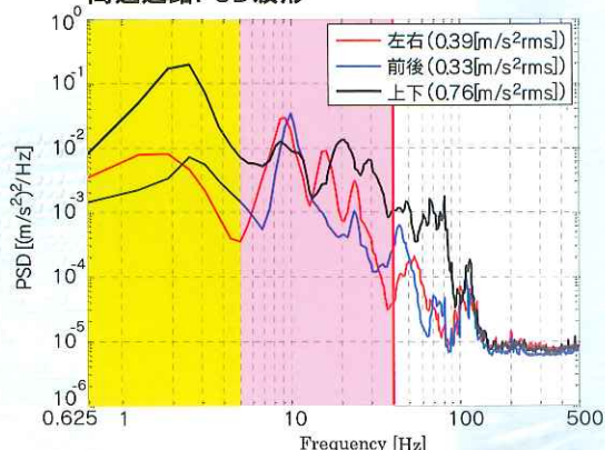
高速道路PSD波形
